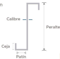
Polín monten tipo “Z”
